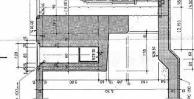
SCHNITT K-K
