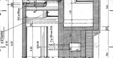
SCHNITT G-G
